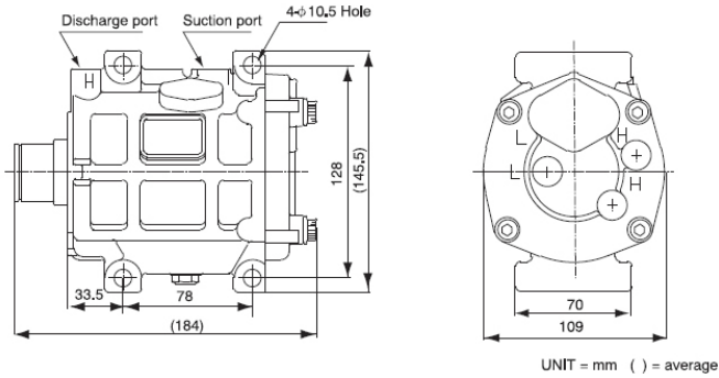
UX120 後出喉管口 (侧视及後视)
