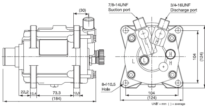
UP120 顶出喉管口(侧视及後视) 安装尺寸同样适用於UPF120
