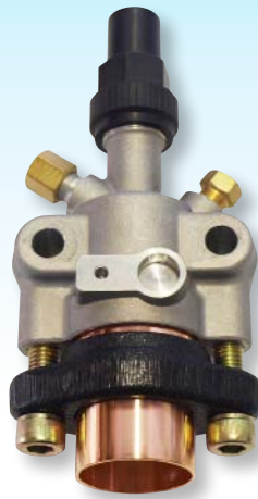
高压注气阀连截止阀 38101-000130
